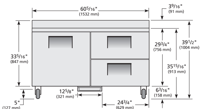
ELEVATION
